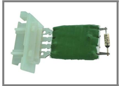
Kalorifer Rezistansı Blower Motor Resistor
