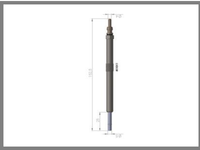
Kızdırma Bujisi Glow Plug MASTER 2.2 2.5 DCI
