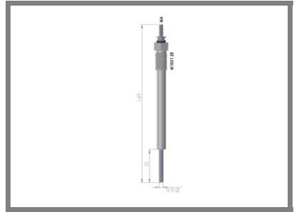
Kızdırma Bujisi Glow Plug H1-STAREX
