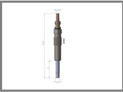
Kızdırma Bujisi Glow Plug CLIO-KANGOO-LAGUNA
