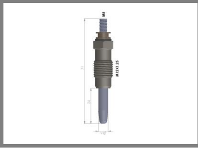
Kızdırma Bujisi Glow Plug AR 6-AR 8 2.4 D
