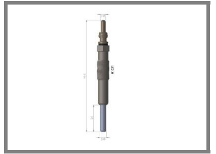
Kızdırma Bujisi Glow Plug CLIO-MEGANE 1.9 D F8Q (00-)
