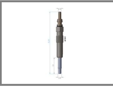
Kızdırma Bujisi Glow Plug A4-A3-A6 1.9 TDI
