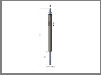
Kızdırma Bujisi Glow Plug MONDEO 1.8 2.0 TDI
