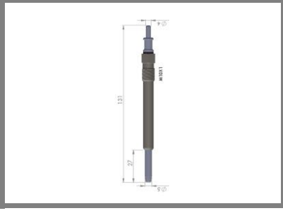
Kızdırma Bujisi Glow Plug C200-E200-SPRINTER
