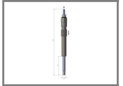
Kızdırma Bujisi Glow Plug JUMPER 2.8 TDI
