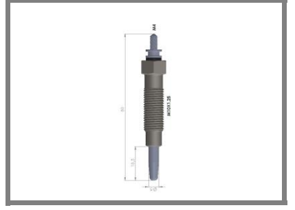
Kızdırma Bujisi Glow Plug L200-L300 2.3D 11V
