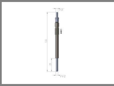
Kızdırma Bujisi Glow Plug FIESTA V-C-MAX-FOCUS II SEDAN 1.4 1.6 TDCI
