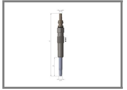
Kızdırma Bujisi Glow Plug A3 1.9 2.0 TDI 5V
