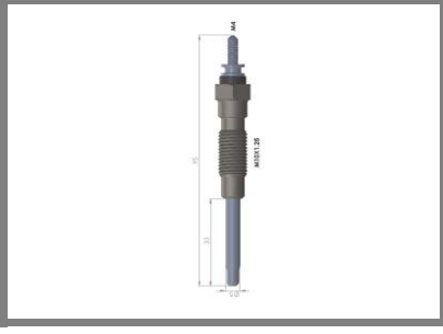
Kızdırma Bujisi Glow Plug HIACE-HILUX PICK UP
