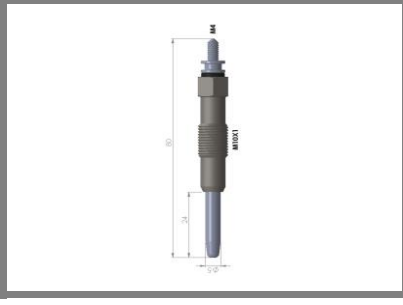
Kızdırma Bujisi Glow Plug DUCATO 2.8 HDI
