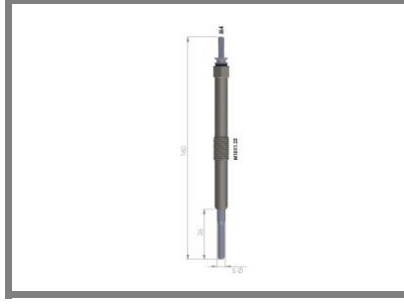
Kızdırma Bujisi Glow Plug YARIS-COROLLA 1.4 D-4D
