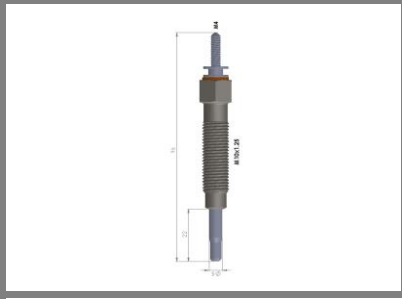
Kızdırma Bujisi Glow Plug L300 (00-02)
