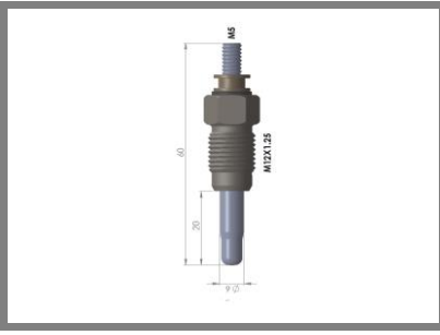
Kızdırma Bujisi Glow Plug 80-100 1.6 2.0 D
