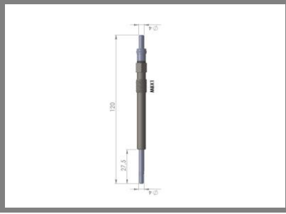
Kızdırma Bujisi Glow Plug DOBLO-PUNTO 1.3
