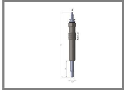
Kızdırma Bujisi Glow Plug CONNECT 1.8 TDCI
