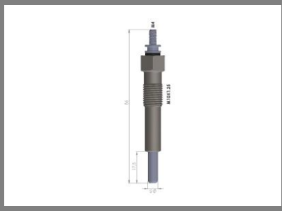
Kızdırma Bujisi Glow Plug COMBO-CORSA 1.5 D
