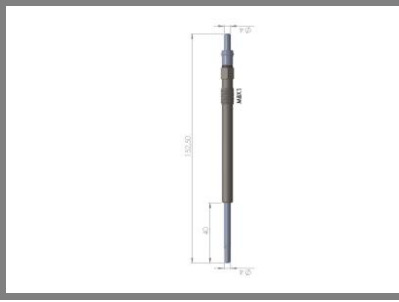
Kızdırma Bujisi Glow Plug DUCATO 2.3 JTD
