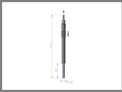
Kızdırma Bujisi Glow Plug FIESTA-FUSION 1.4 TDCI
